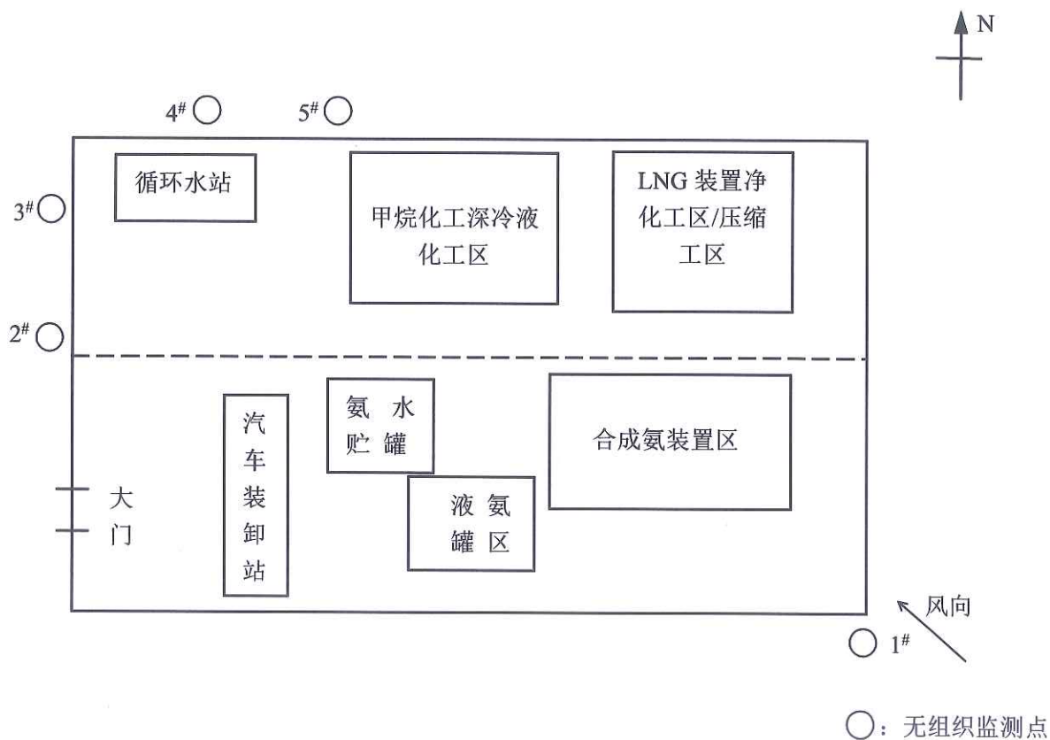
图 4-2 厂界无组织监测点位示意图
