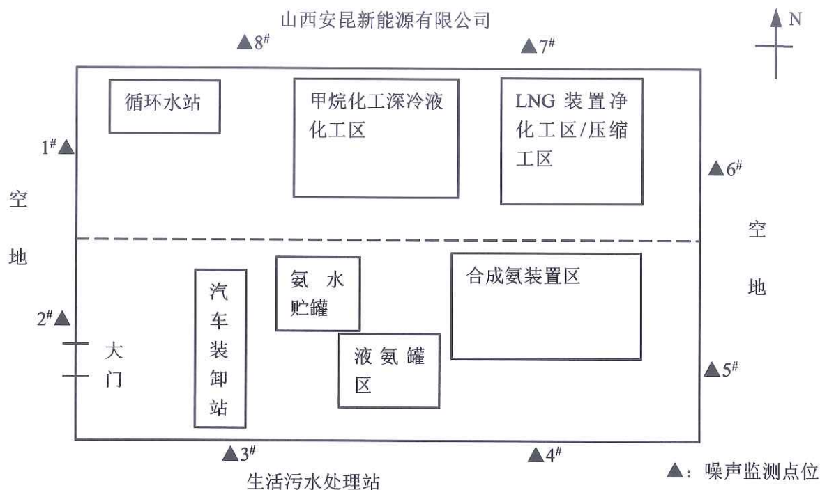
图 4-3 厂界噪声监测点位示意图
