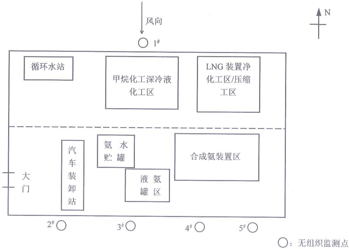
图 4-2 厂界无组织监测点位示意图
