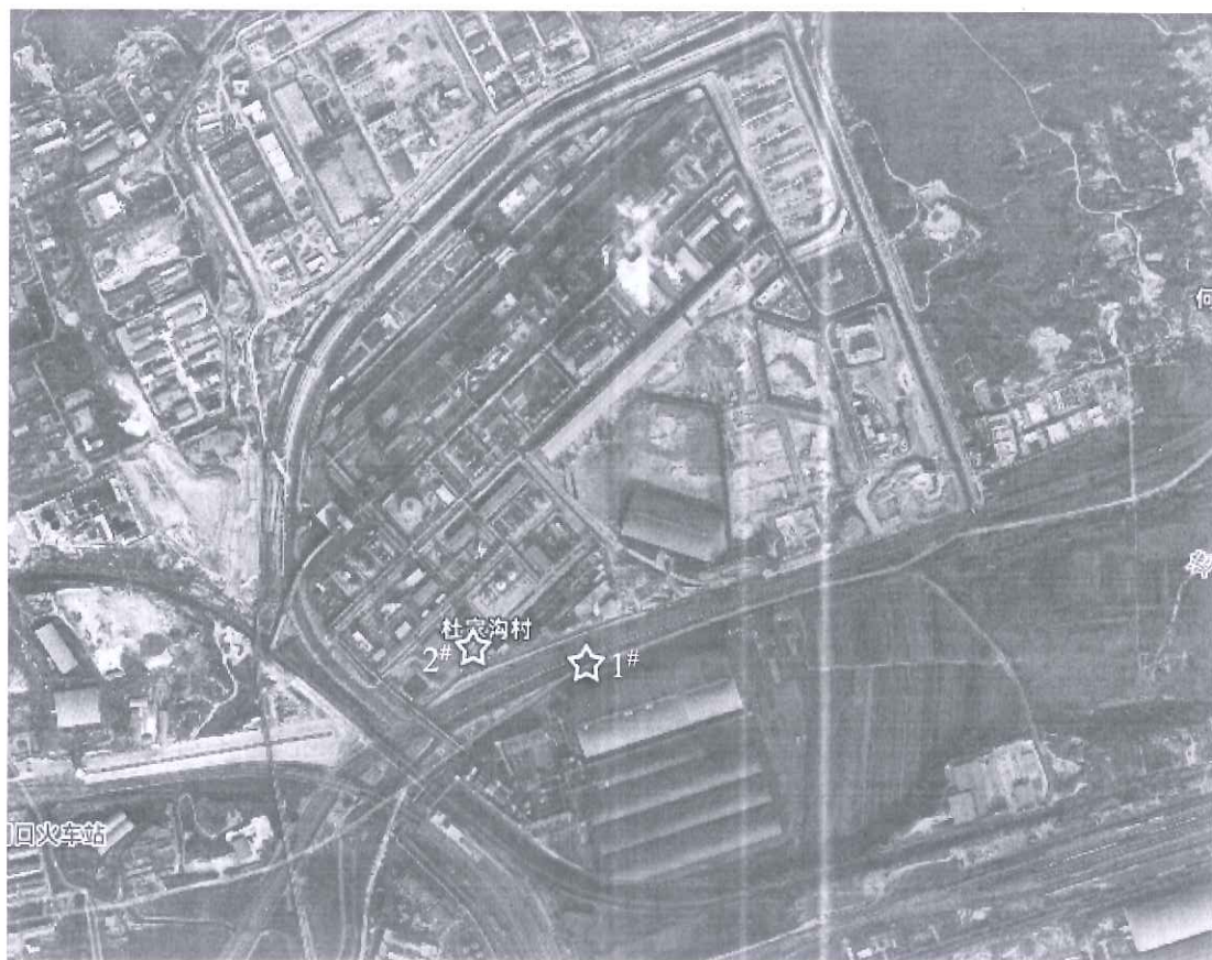
图 4-1 地下水监测点位平面示意图
