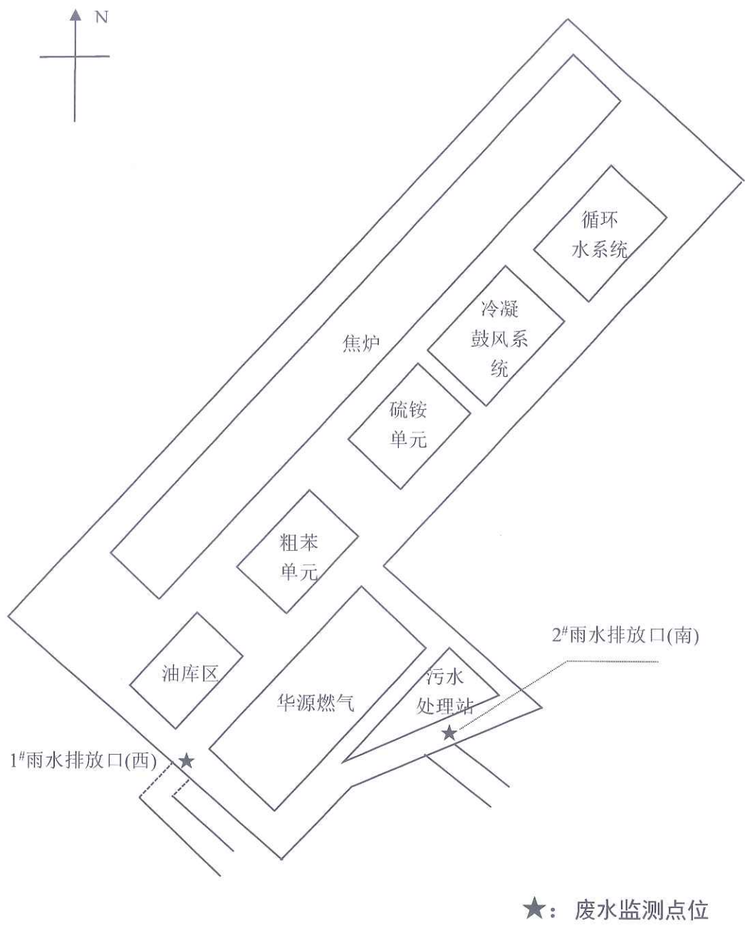
图 4-1 雨水排放口监测点位平面示意图
