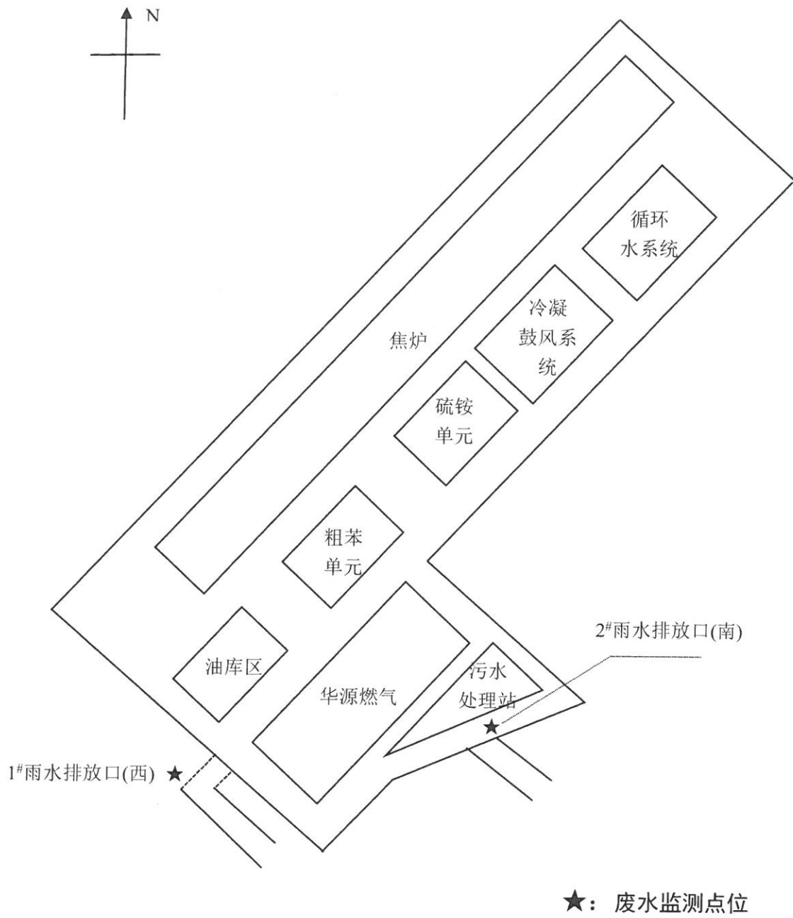
图 4-1 雨水排放口监测点位平面示意图
