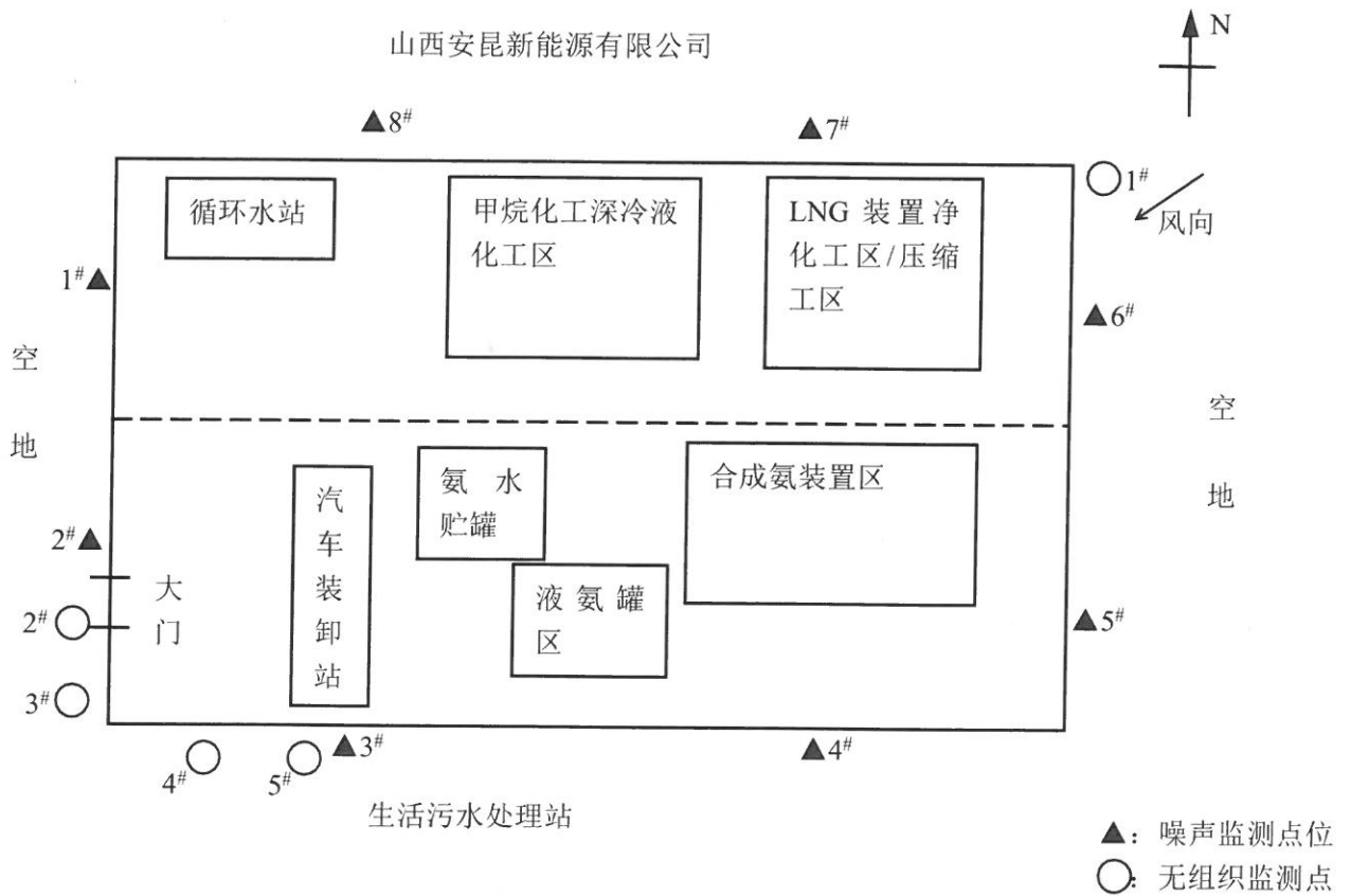
图 4-2 厂界无组织及噪声监测点位示意图
