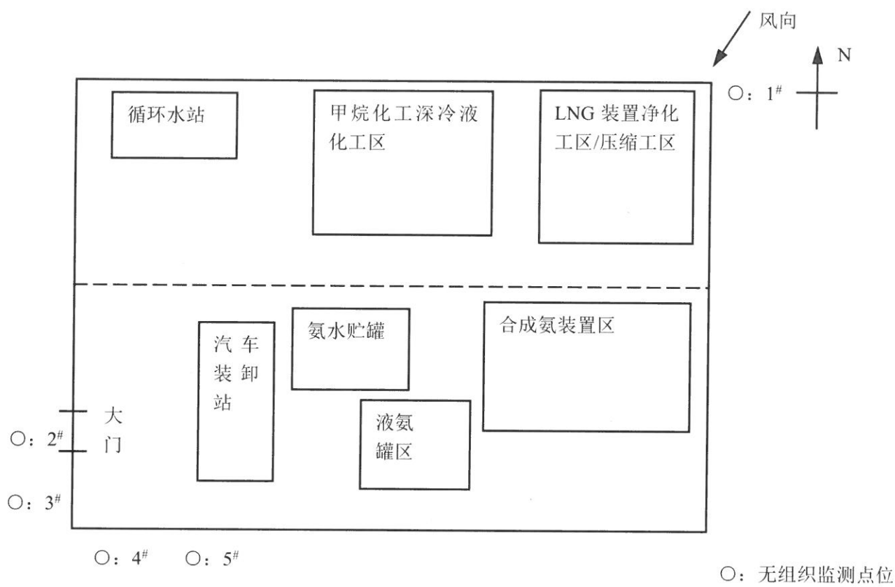
图 4-2 厂界无组织监测点位示意图（07 月 25 日）
