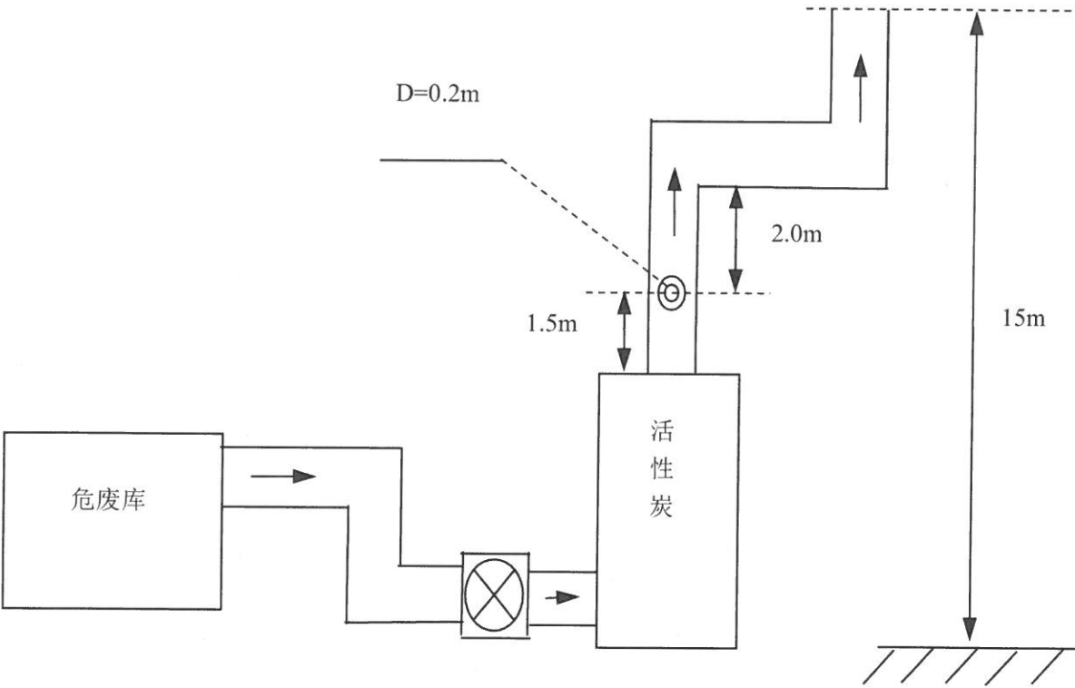
图 4-1 危废库监测点位示意图（07 月 25 日）
