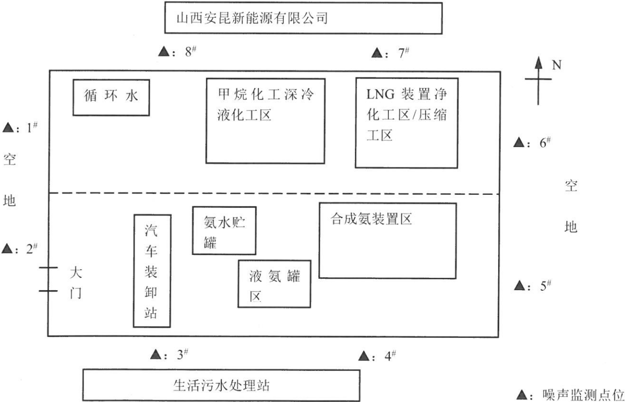
图 4-3 厂界噪声监测点位示意图（09 月 02 日）
