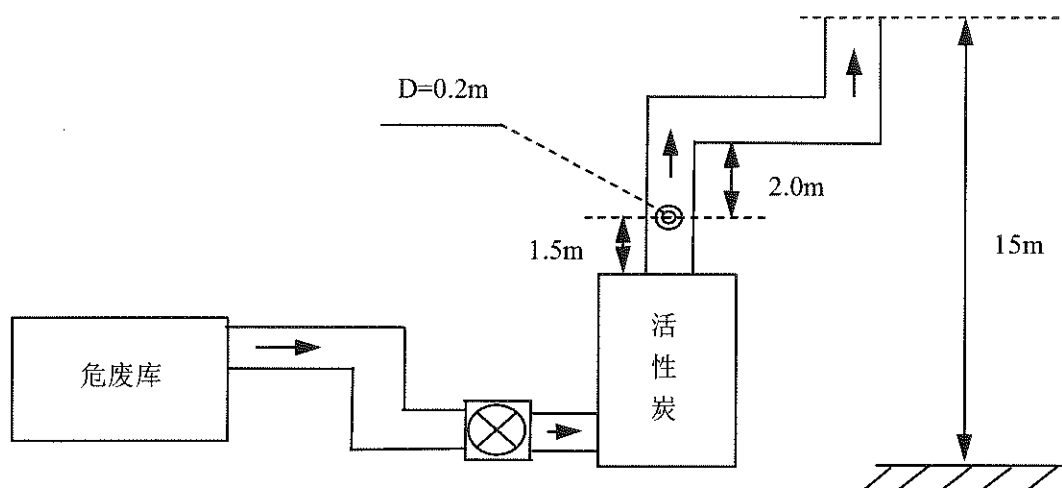
图 4-3 危废库监测点位示意图（6 月 9 日）
