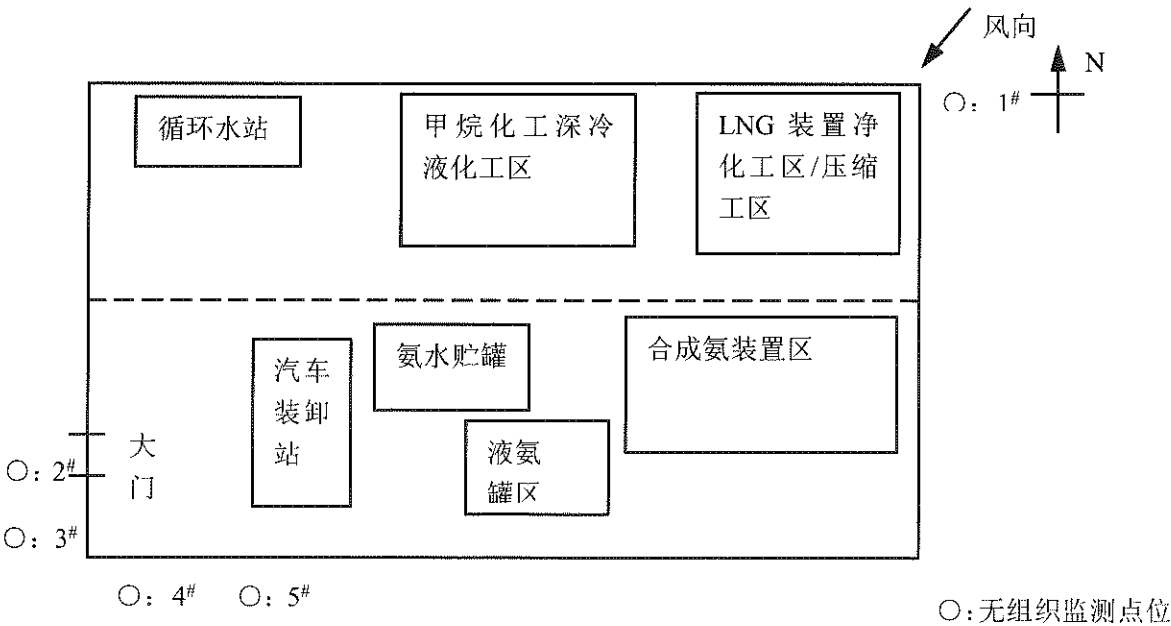
图 4-1 厂界无组织监测点位示意图（5 月 29 日）
