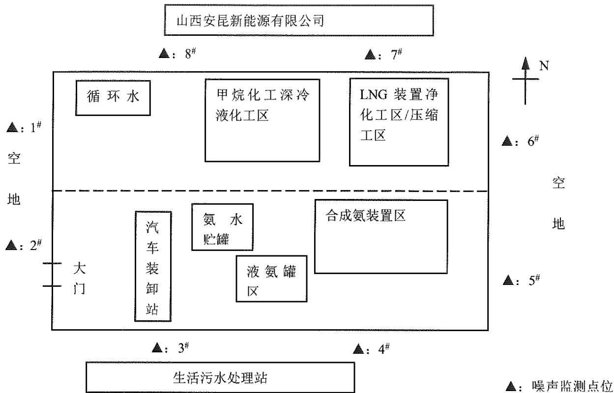
图 4-2 厂界噪声监测点位示意图（5 月 15 日）
