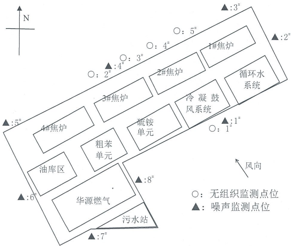
图 4-12 厂界噪声、厂界无组织监测点位平面示意图
