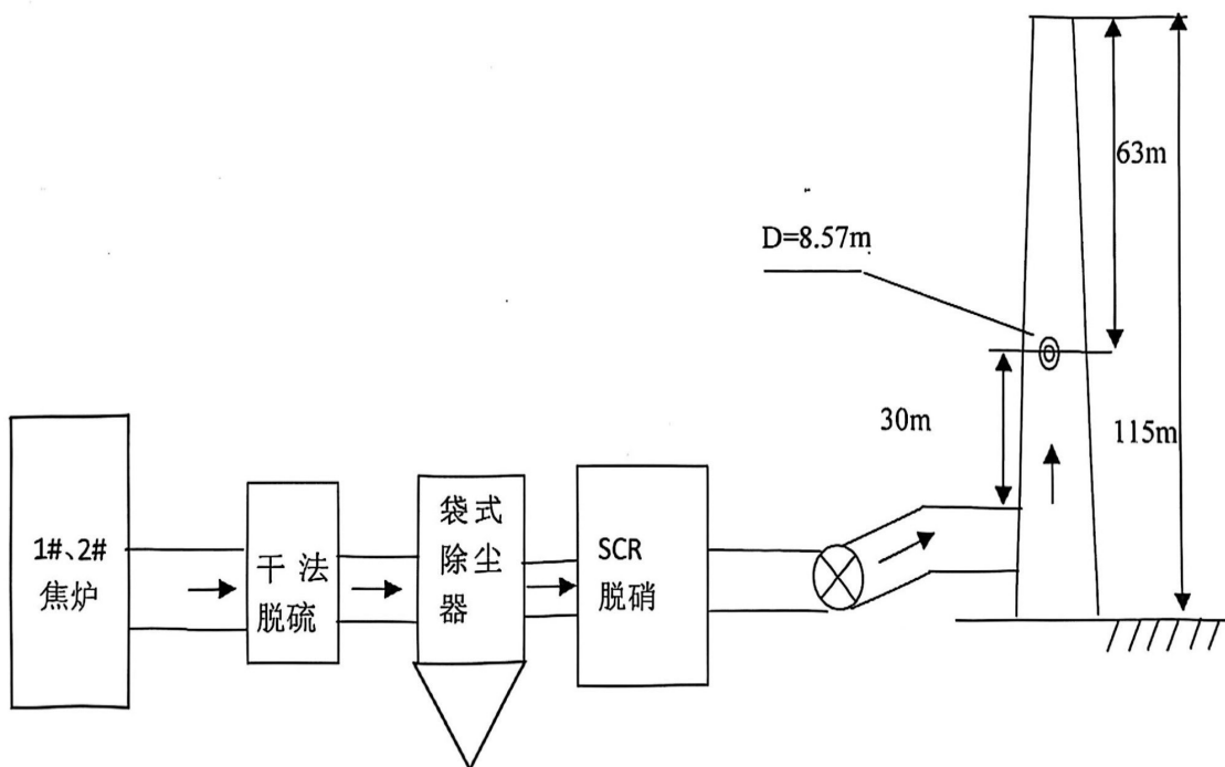
图 3-8 1#焦炉烟囱监测点位示意图
