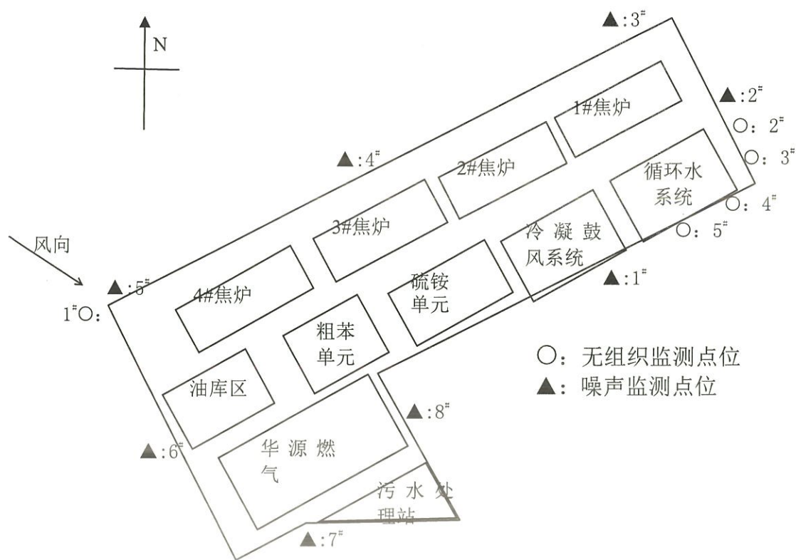
图 4-5 厂界噪声、厂界无组织监测点位平面示意图
