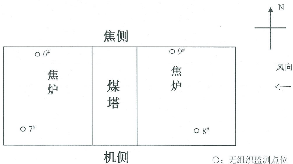
图 4-2 焦炉炉顶无组织监测点位示意图
