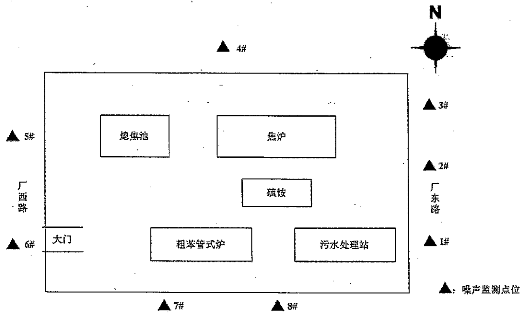
图 4-3 噪声监测点位示意图
