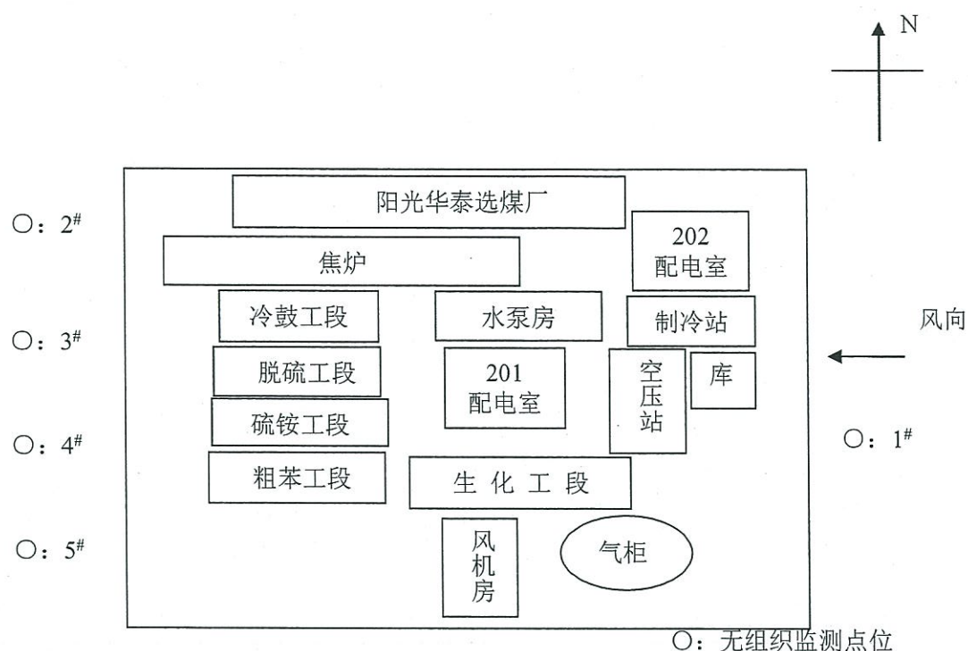
图 4-1 厂界无组织监测点位示意图
