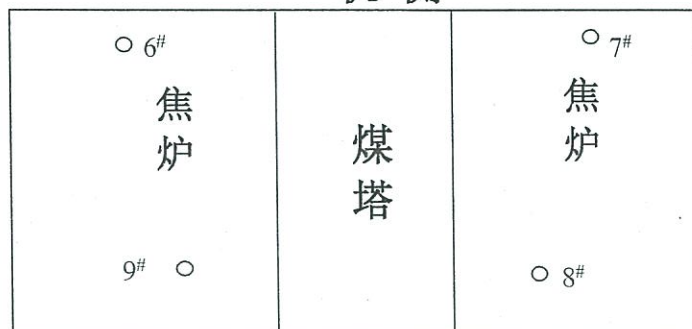
图 4-2 焦炉炉顶无组织监测点位示意图
