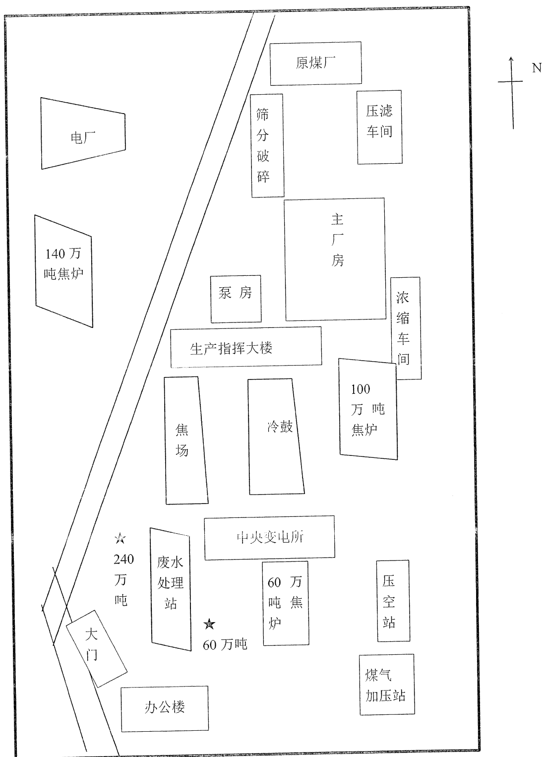
图1 污水监测点位平面示意图
