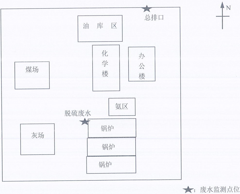
图 4-1 厂区废水总排口监测点位示意图
