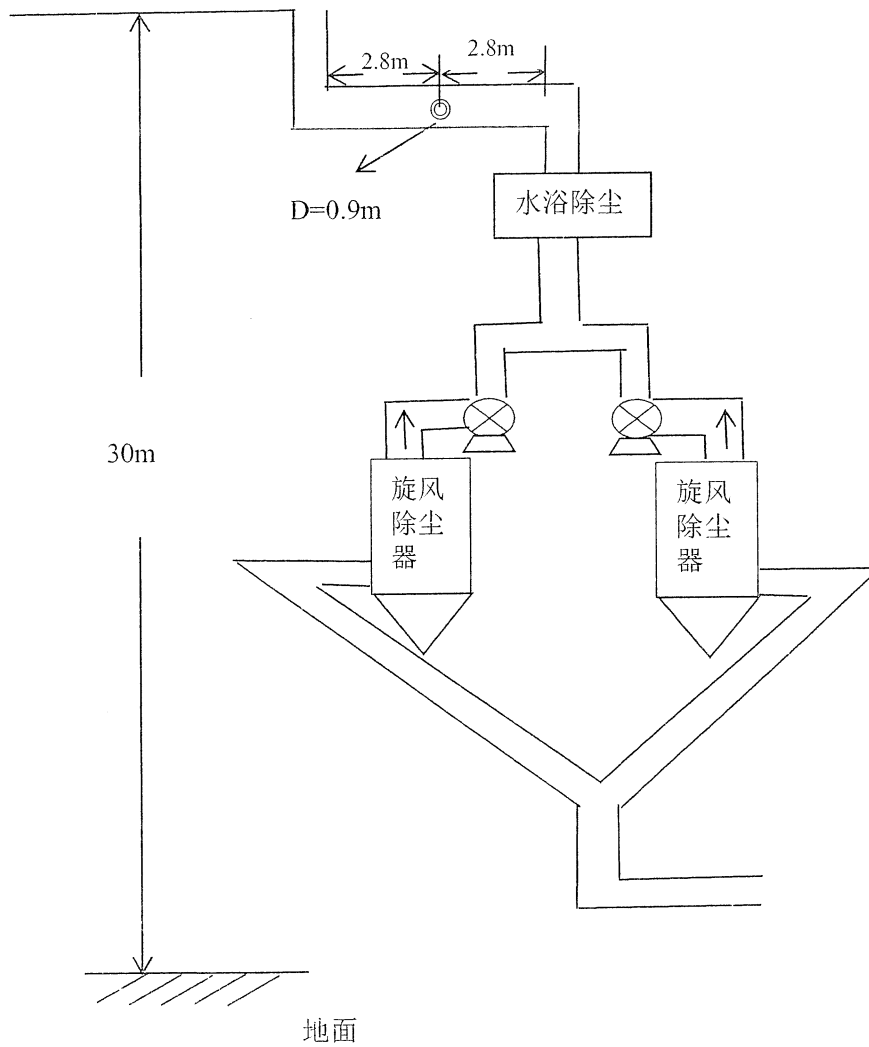
图 4-3 100 万、60 万、140 万硫铵合用除尘器监测点位
