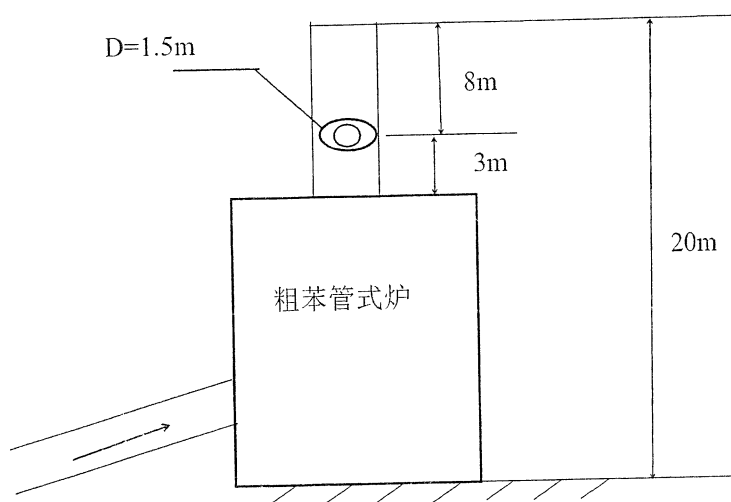
图 4-1 1#、2#粗苯管式炉监测点位示意图
