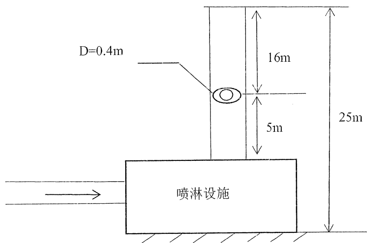
图 4-3 油库洗净塔监测点位示意图
