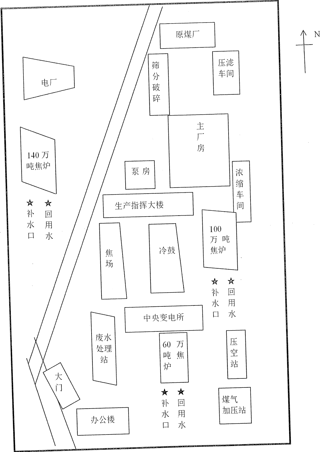
图 1 污水监测点位平面示意图
